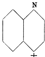
Naphthionsäure. (Piria.)
